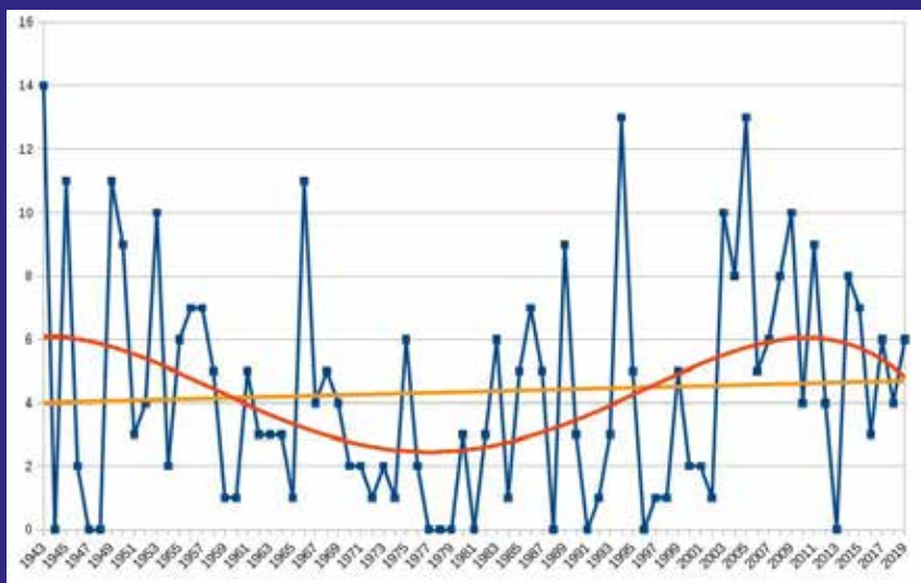
Gràfic de l'evolució de les nits tropicals a Atzeneta des del 1943 fins al 2019. Amb taronja la tendència ajustada a una funció lineal i amb roja la tendència ajustada a una funció polinòmica.
